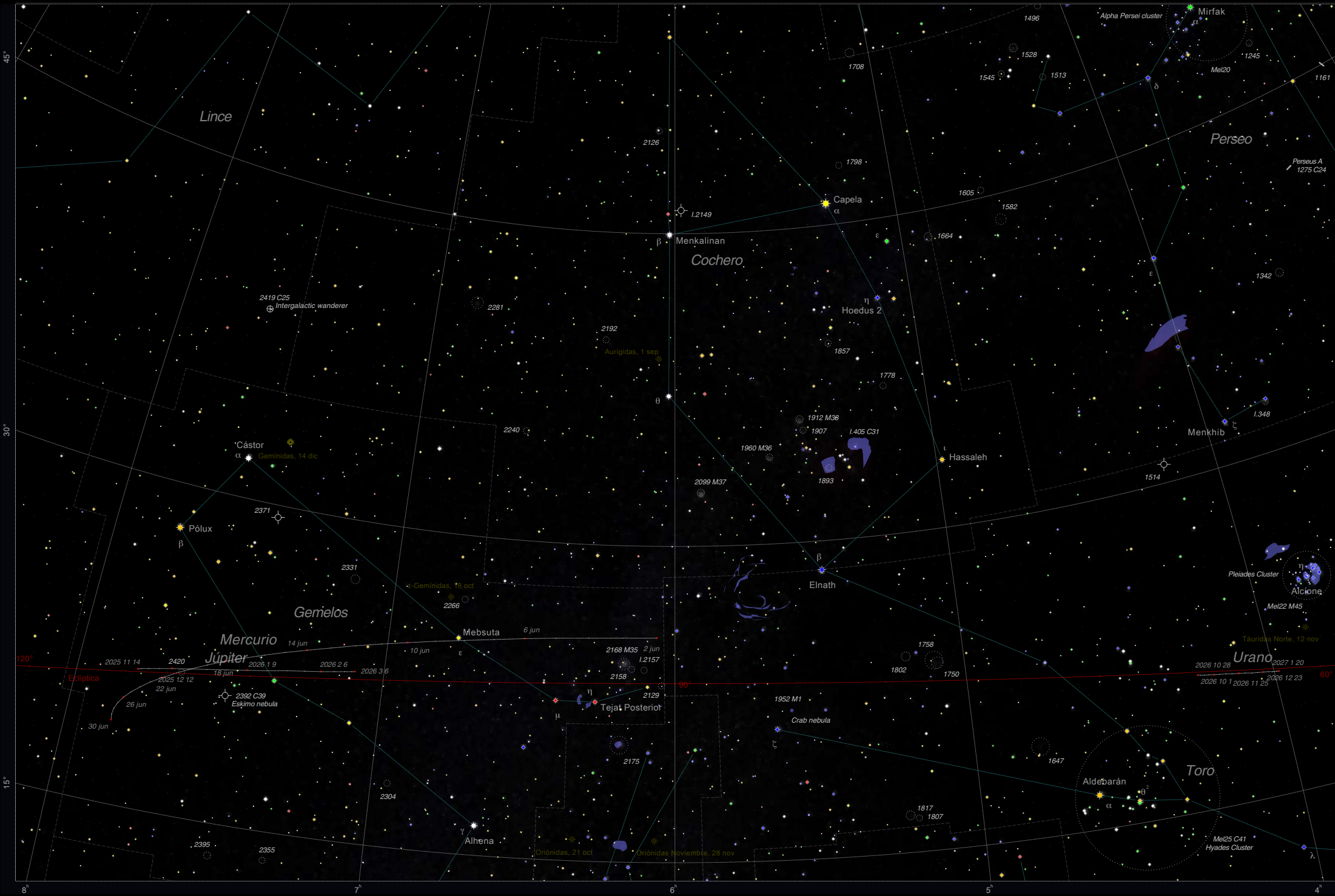
Carta 5, 30°×20° alrededor de 6.0h, 35.0° (Cochero, Gemelos, Toro, Orión)
