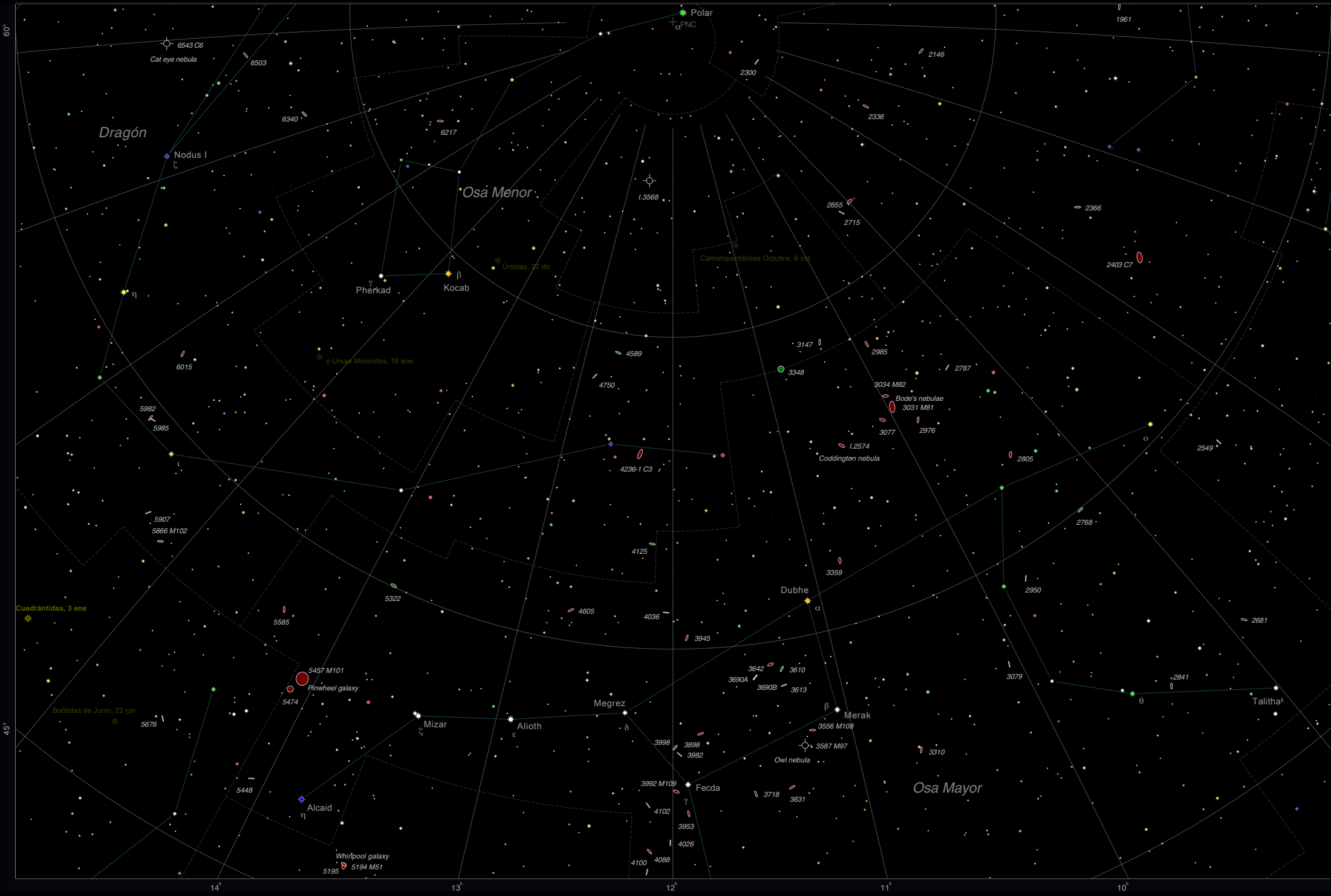
Carta 2, 30°×20° alrededor de 12.0h, 70.0° (Dragón, Osa Mayor, Osa Menor, Jirafa)
