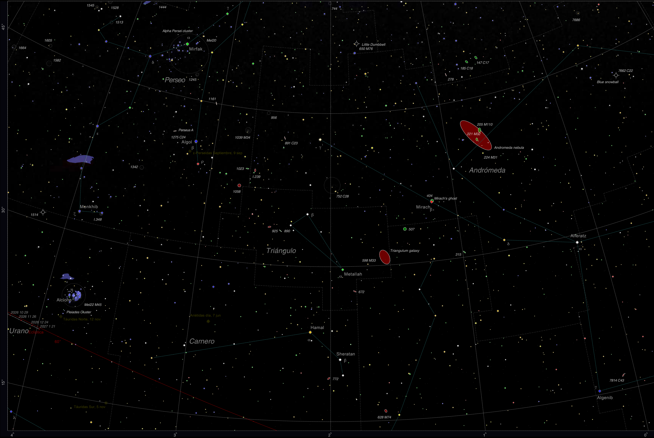
Carta 4, 30°×20° alrededor de 2.0h, 35.0° (Triángulo, Andrómeda, Perseo, Peces)
