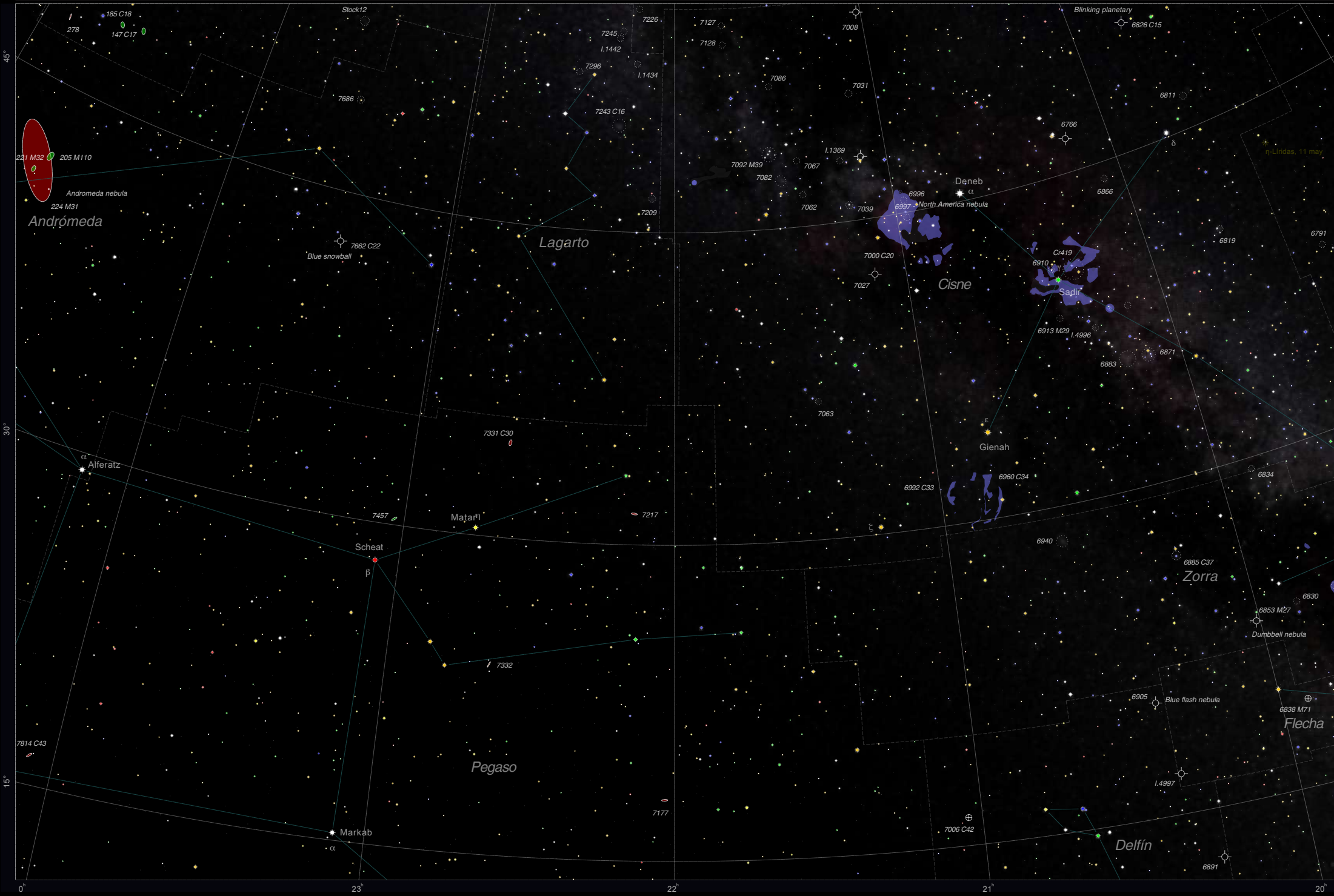
Carta 9, 30°×20° alrededor de 22.0h, 35.0° (Pegaso, Lagarto, Cisne, Zorra)
