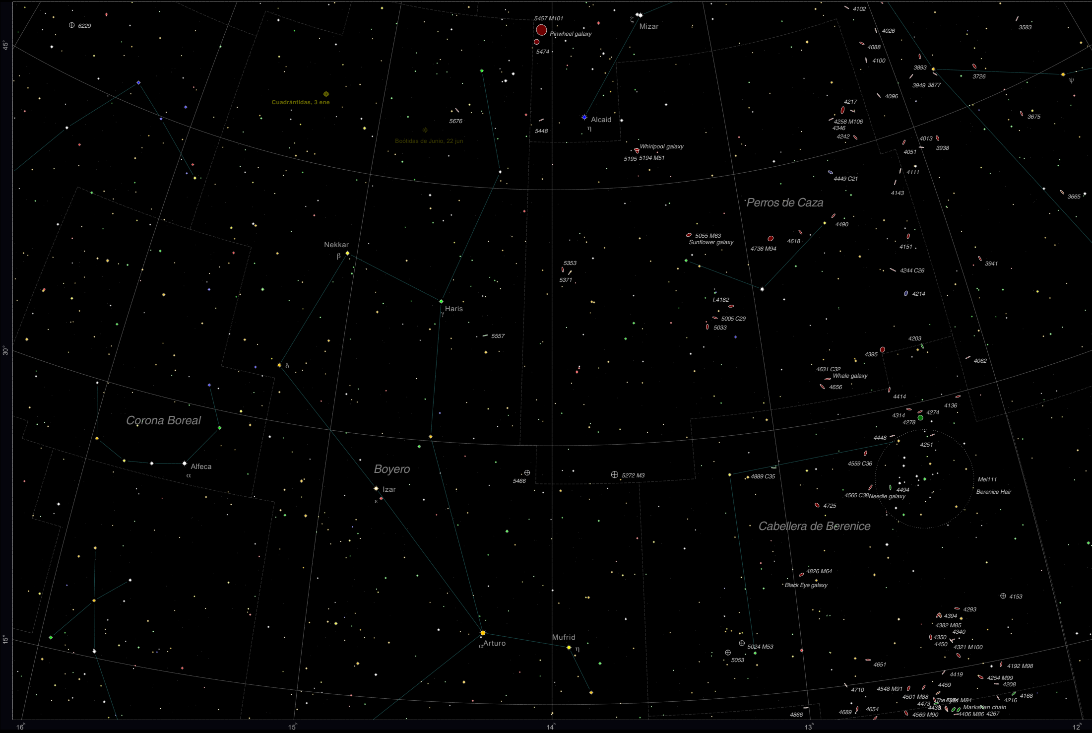
Carta 7, 30°×20° alrededor de 14.0h, 35.0° (Perros de caza, Boyero, Osa Mayor, Cabellera de Berenice)
