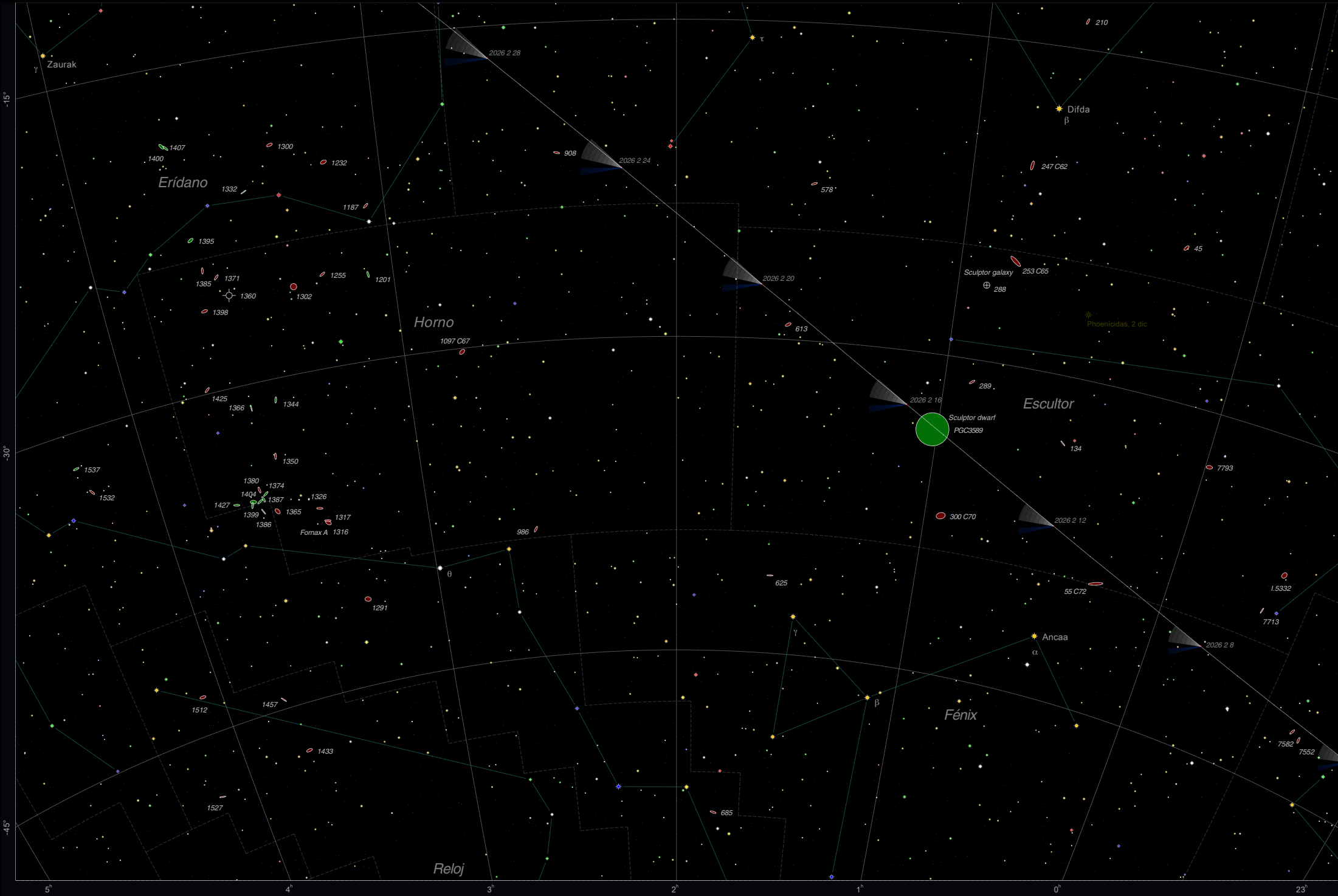
Carta 18, 30°×20° alrededor de 2.0h, -35.0° (Horno, Escultor, Fénix, Ballena)
