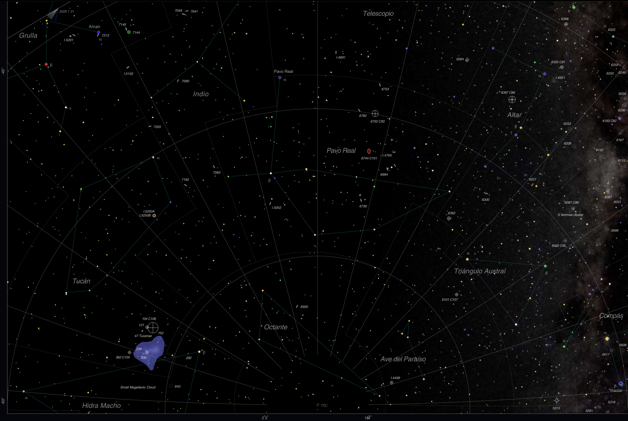
Carta 26, 30°×20° alrededor de 20.0h, -70.0° (Pavo Real, Octante, Indio, Telescopio)
