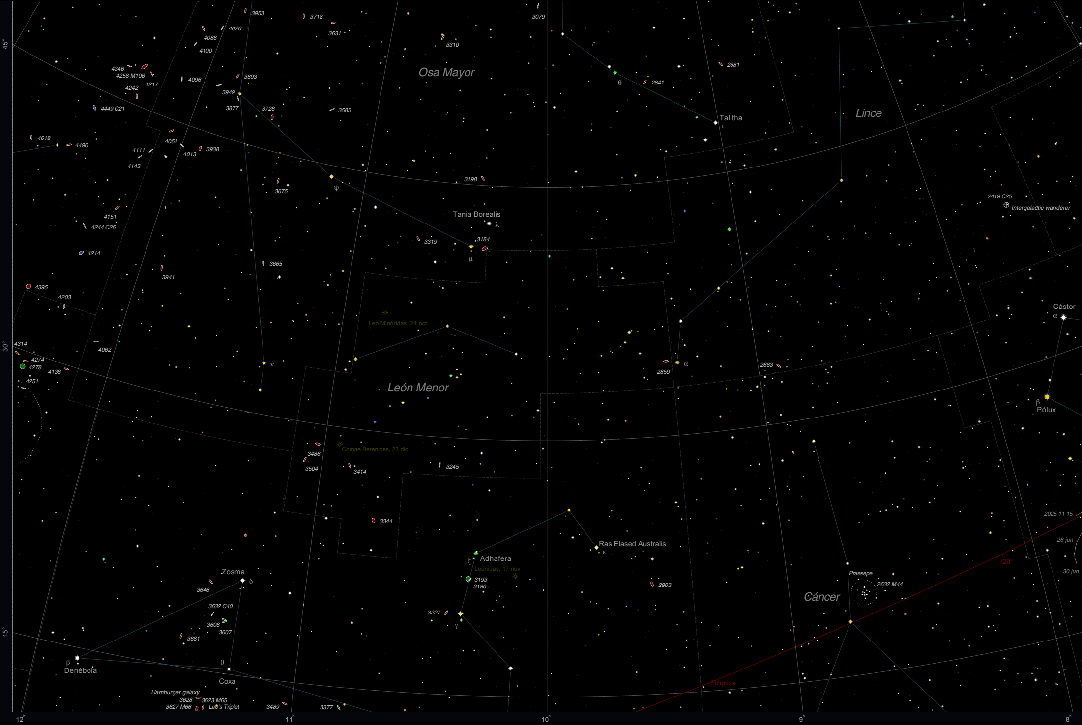
Carta 6, 30°×20° alrededor de 10.0h, 35.0° (León Menor, Osa Mayor, Lince, Cáncer)
